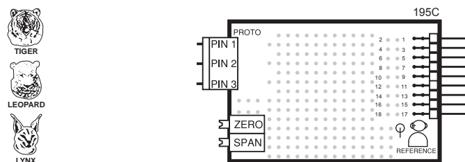
IR02: 3 wire Potentiometer 1K \Omega min (0- \infty .)
