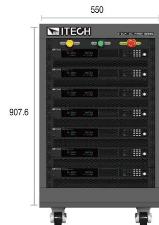
IT-E4029-15U (Dimension:mm)
