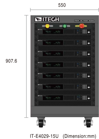
IT-E4029-15U (Dimension:mm)
